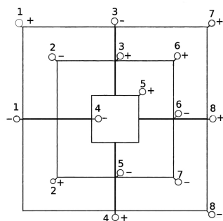
სწორი დიუზის ფორმა და ქვების განლაგება
